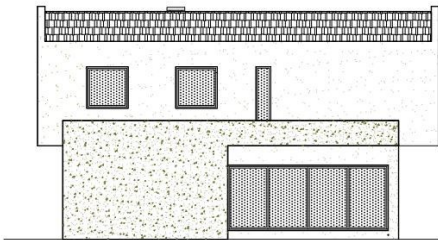
SJEVEROZAPADNO PROČELJE
