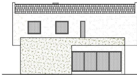
SJEVEROZAPADNO PROČELJE
