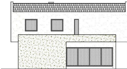
SJEVEROZAPADNO PROČELJE
