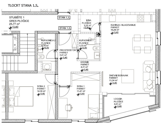
POVRŠINA STANA 1.5.
