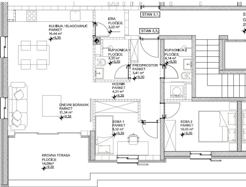
TLOCRT STANA 3.3.
