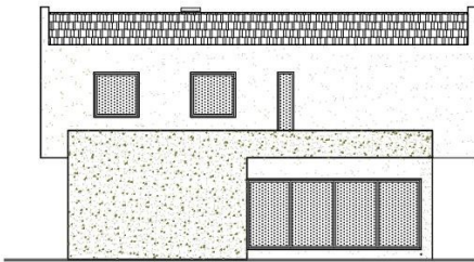
SJEVEROZAPADNO PROČELJE
