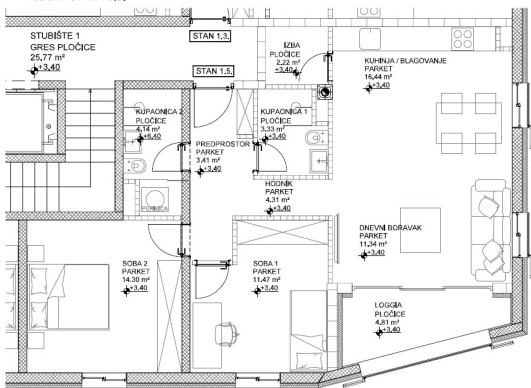
TLOCRT STANA 1.5.
